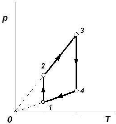
Рис. 1. График изопроцессов в координатах pT
